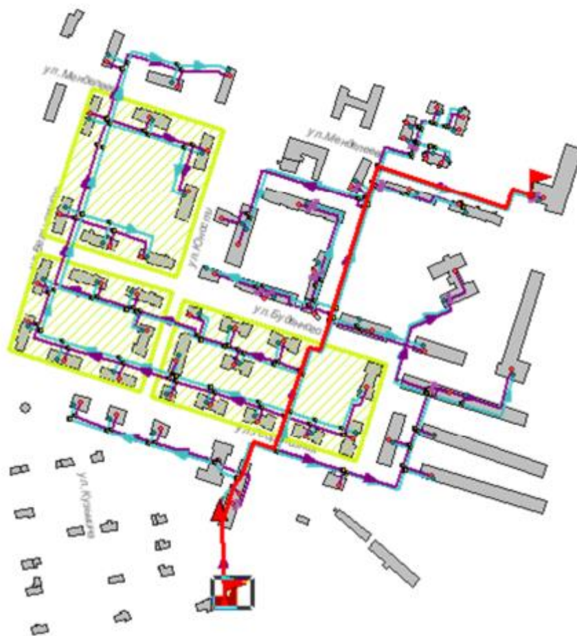
Рисунок 31.3 -Расчетный путь теплоносителя от котельной до Менделеева,19
