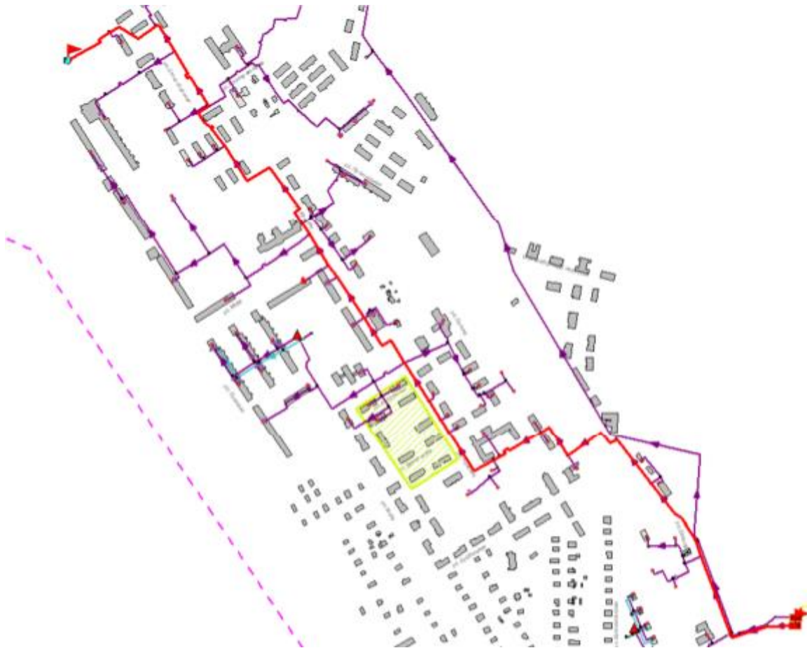
Рисунок 2.3 -Расчетный путь теплоносителя от Цигломенской ТЭС до Лочехина, д.13
