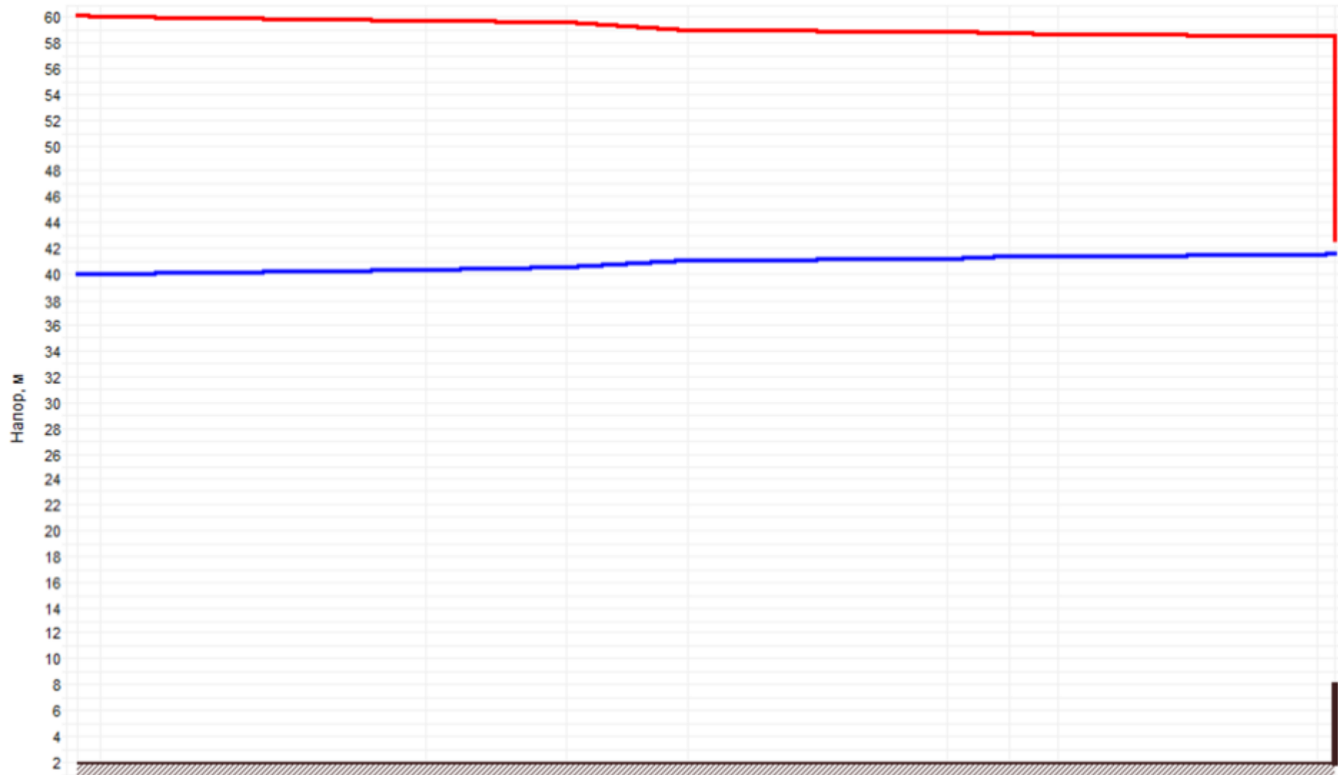
Рисунок 32.2 –График гидравлических режимов рассматриваемого теплопровода
