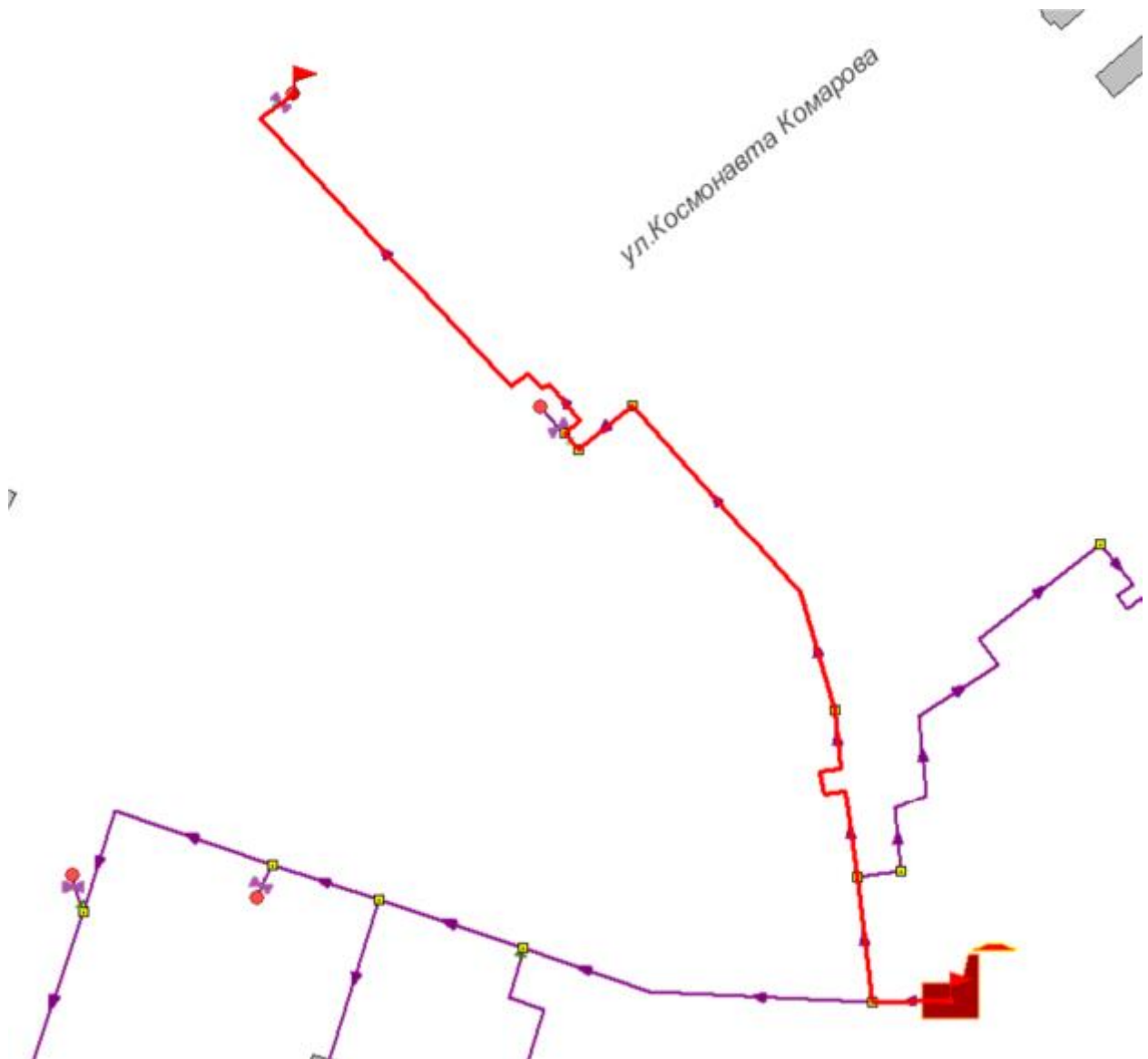
Рисунок 35.3 -Расчетный путь теплоносителя от котельной до Комарова, 14
