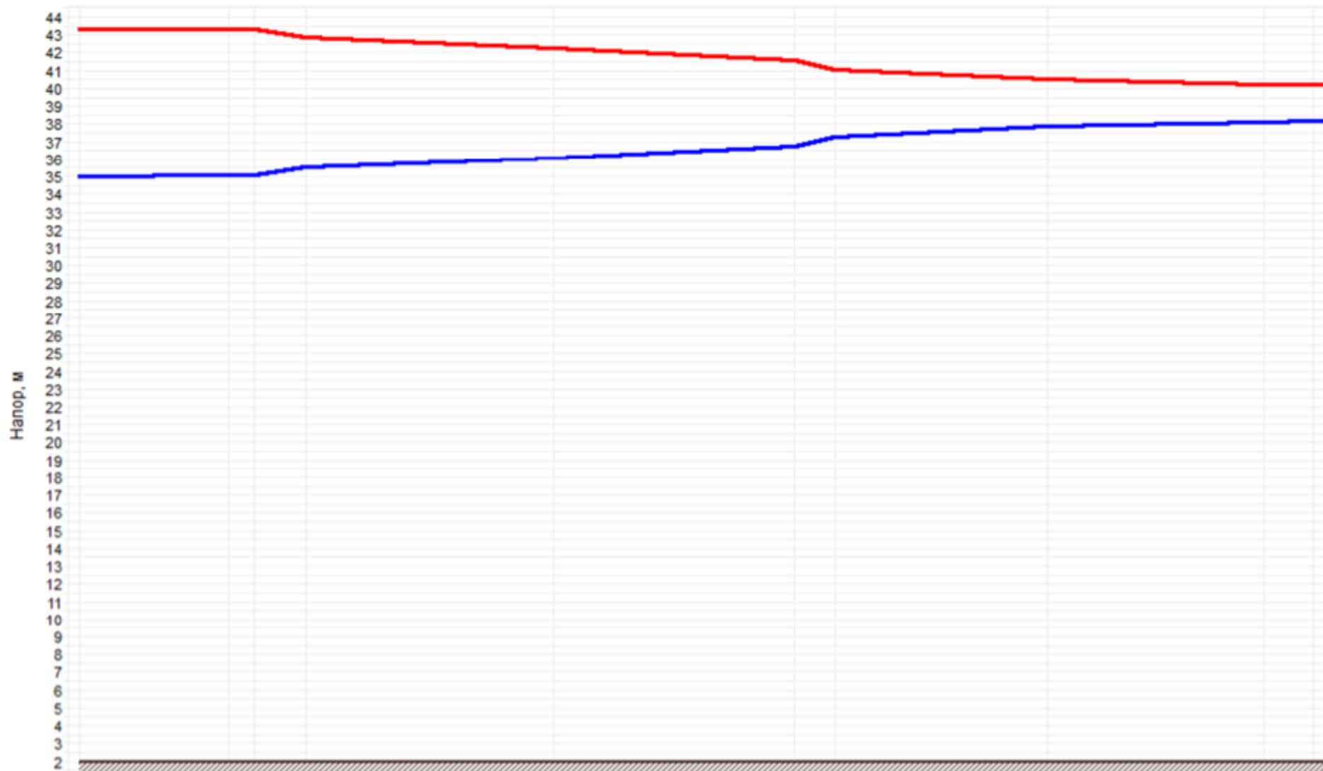
Рисунок 20.2 –График гидравлических режимов рассматриваемого теплопровода
