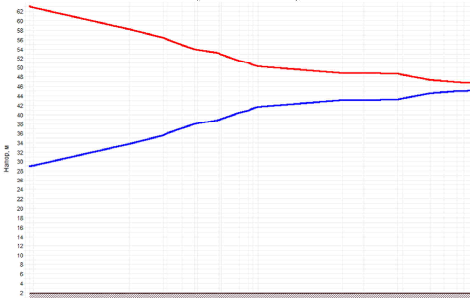
Рисунок 10.2 –График гидравлических режимов рассматриваемого теплопровода
