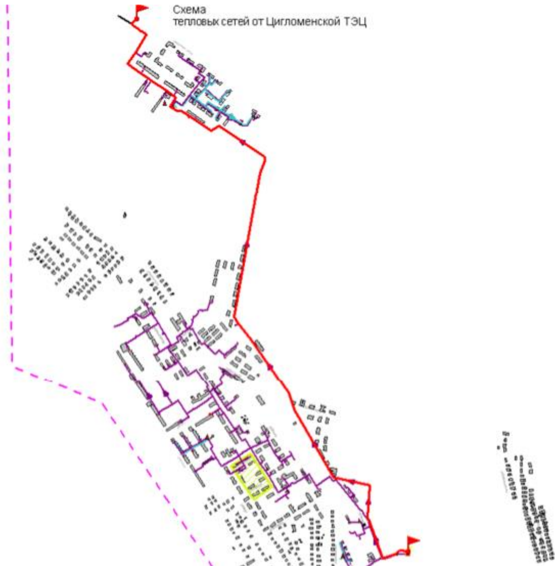
Рисунок 2.1 -Расчетный путь теплоносителя от Цигломенской ТЭС до кирпичного завода
